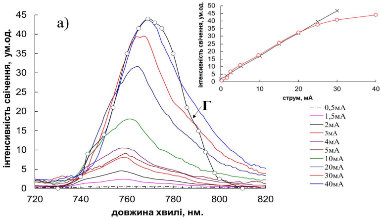
Рис. 5 (а) Червона смуга випромінювання УФ світлодіода T = 300 К, Г – розподіл Гауса (-o-). На вставці показана залежність інтенсивності випромінювання від струму (x- розрахунок, -o- експеримент)
