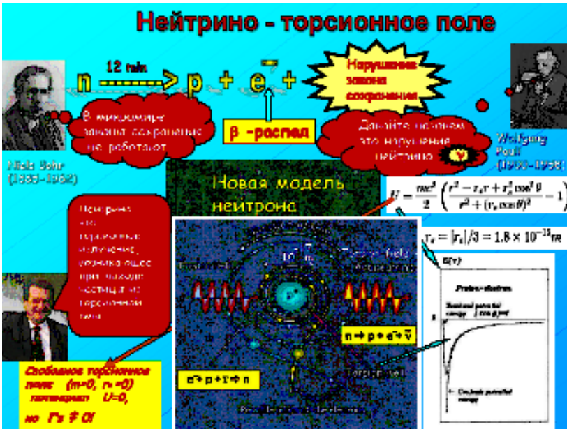
Рис. 7. Модель нейтрона, следующая из уравнений Физического Вакуума
