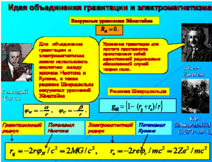
Рис. 4. Объединение гравитационных и электромагнитных взаимодействий
